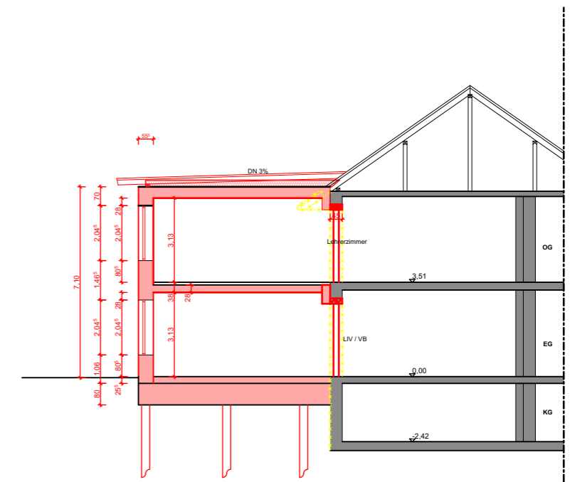
Schnitt Entwurf
